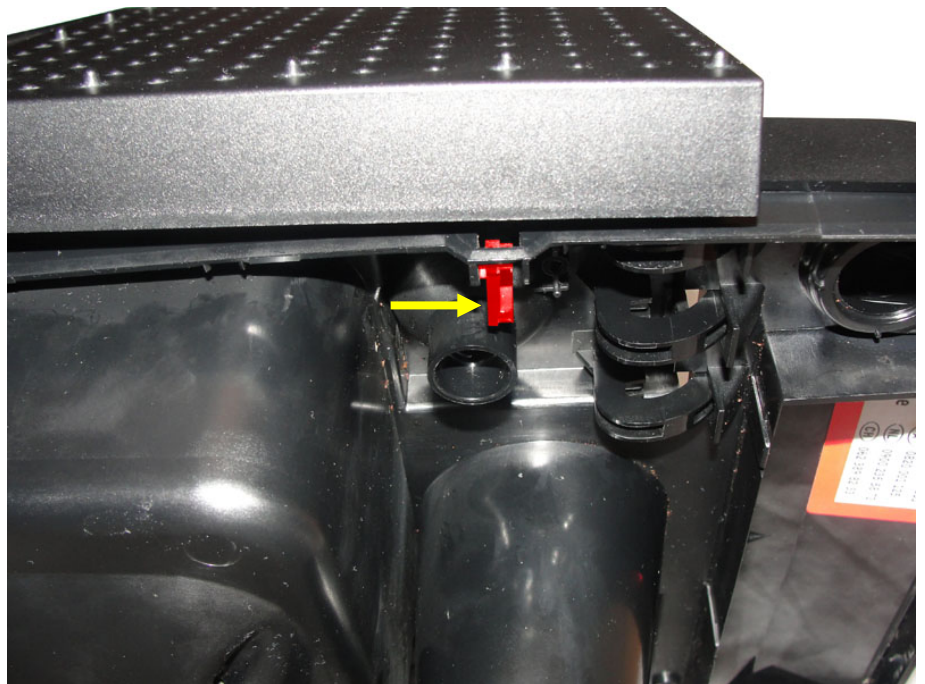
rechtes Scharnier
